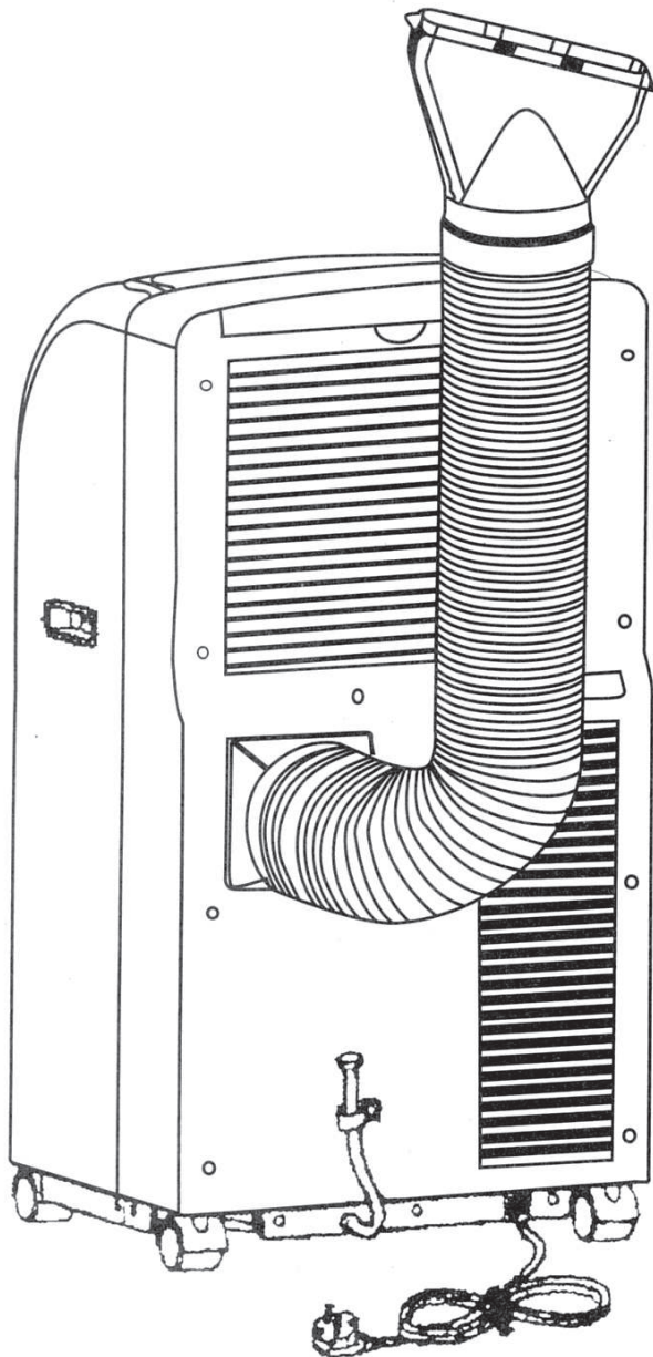
Bild 4: Montage des Abluftschlauchs
